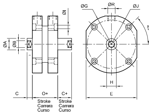
Ø 20...100 doble vástago
