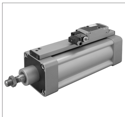
Serie CN10 + Namur
