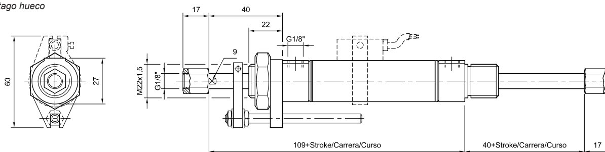
Vástago hueco con amortiguación
