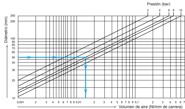
Ávaco para el cálculo del volúmen de aire por mm de carrera
